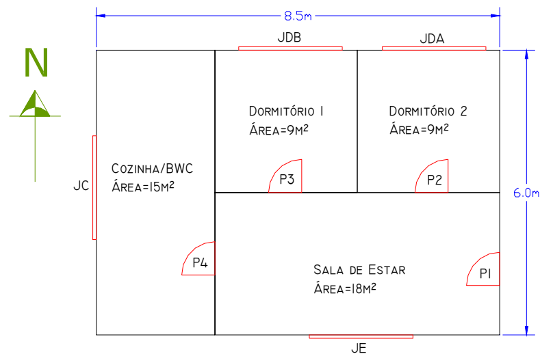
Figura 1. Vista em planta do modelo simulado.
